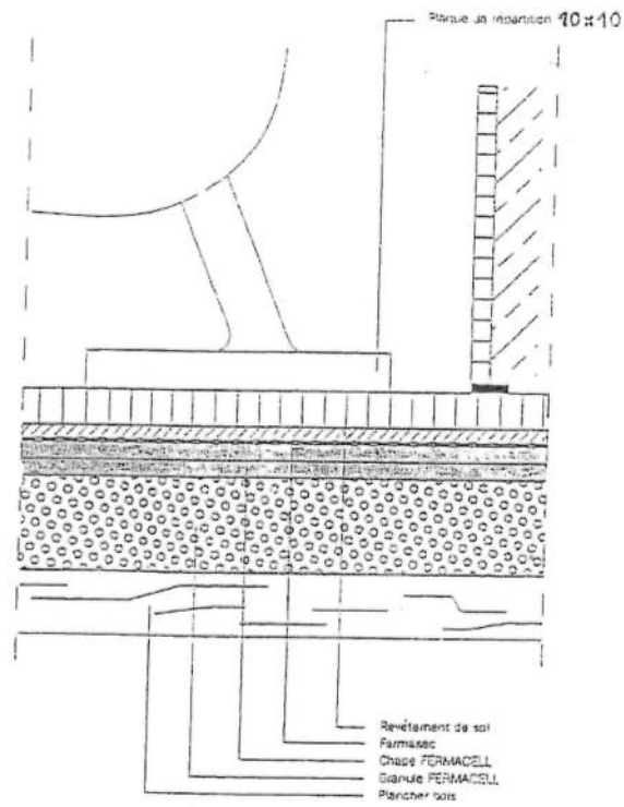
Figure 14 – Pose de baignoire
