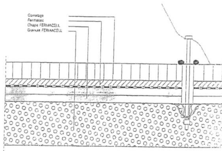
Figure 15 – Fixation des appareils sanitaires
